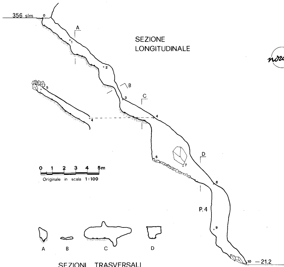
SEZIONI TRASVERSALI
